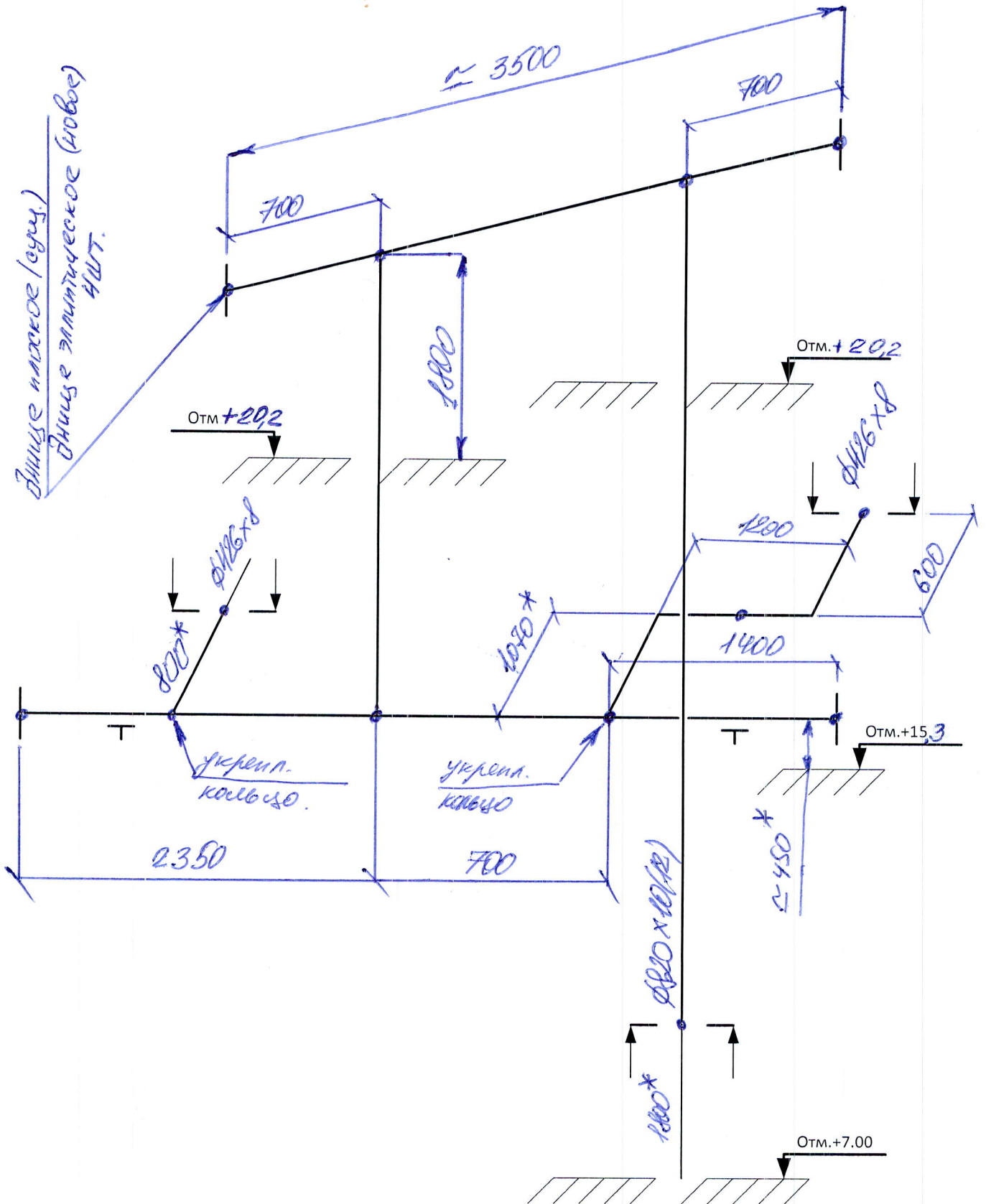
Схема участка газохода реакционного газа после реактора P-101/1 в T-101/3а,б
