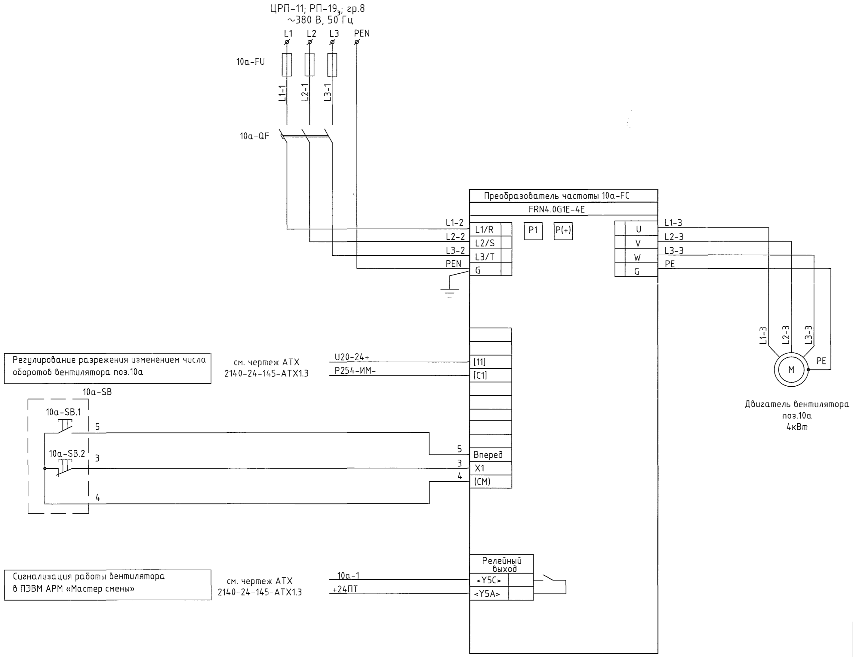
Принципиальная схема управления электродвигателем вентилятора поз.10а
