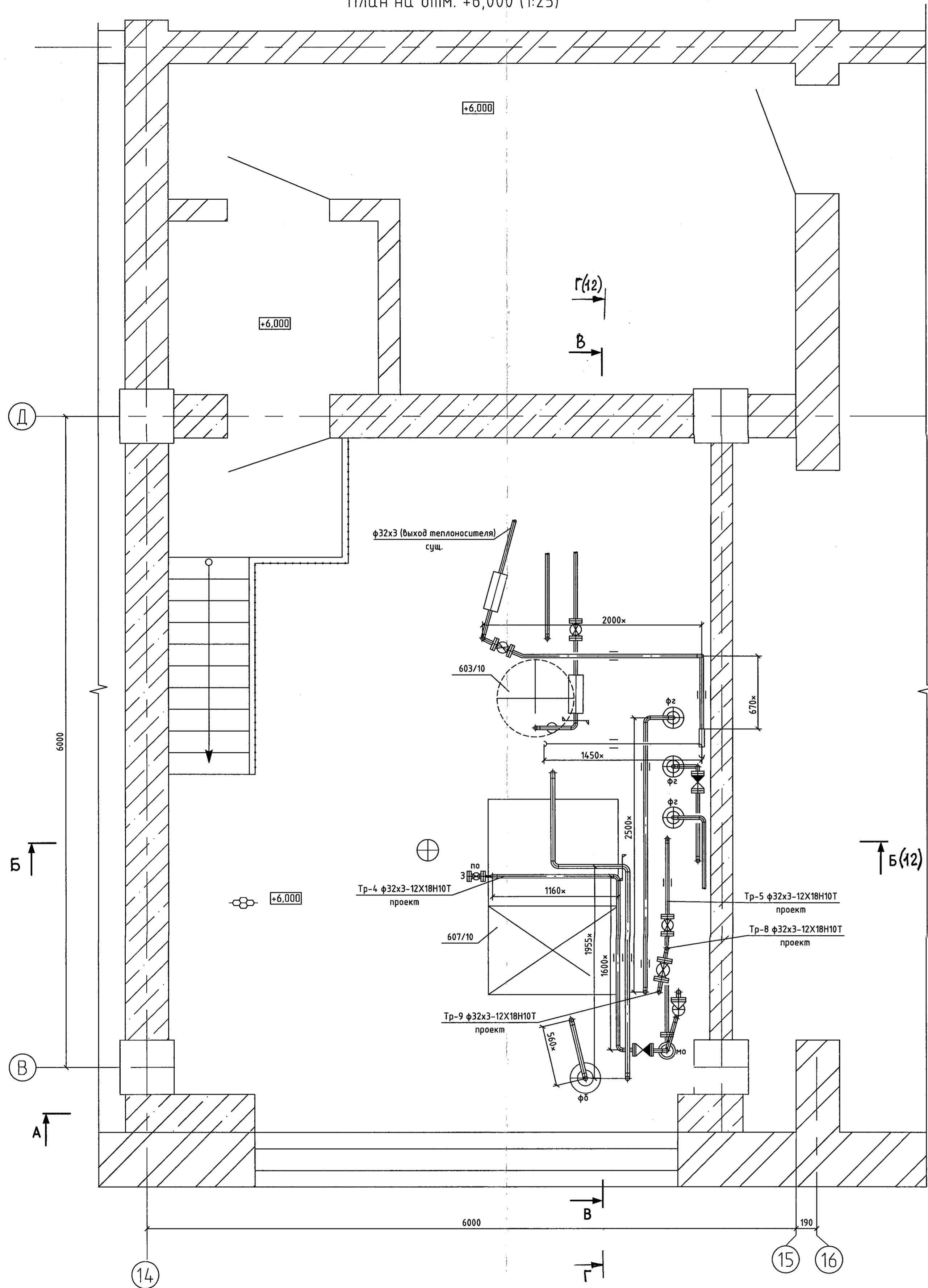
План на отм. +6,000 (1:25)
