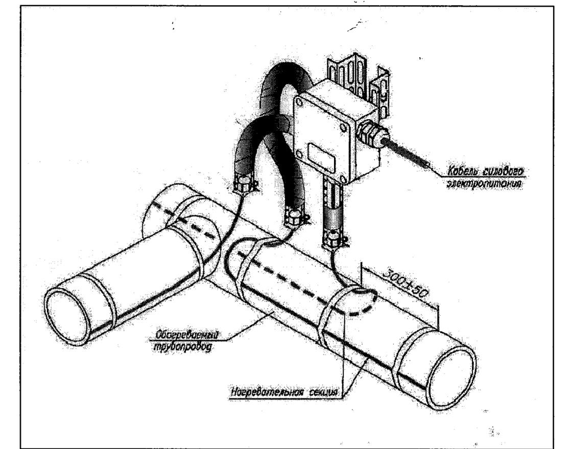
Подвод питания к саморегулирующим нагревательным лентам
