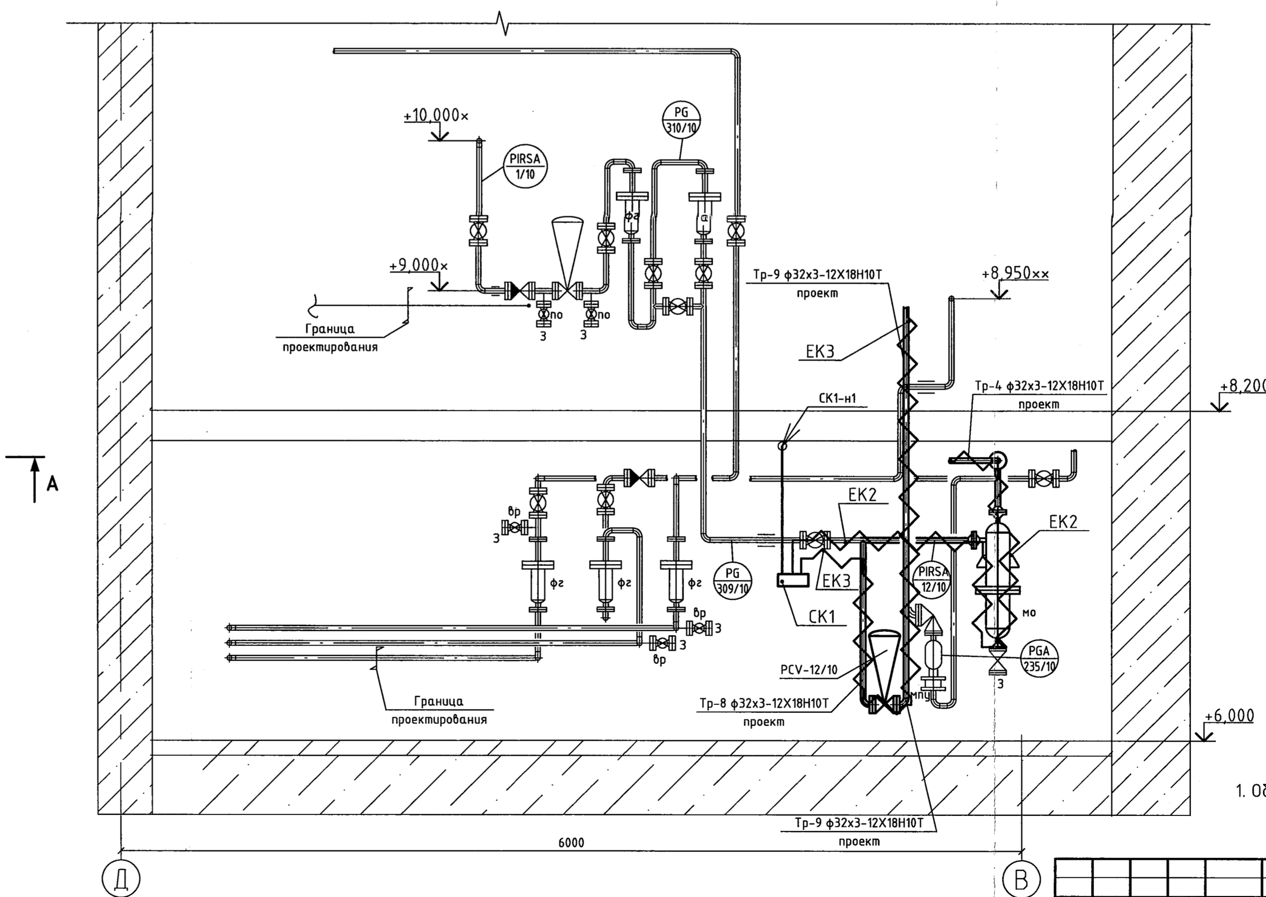
Разрез В-В (1:25)
