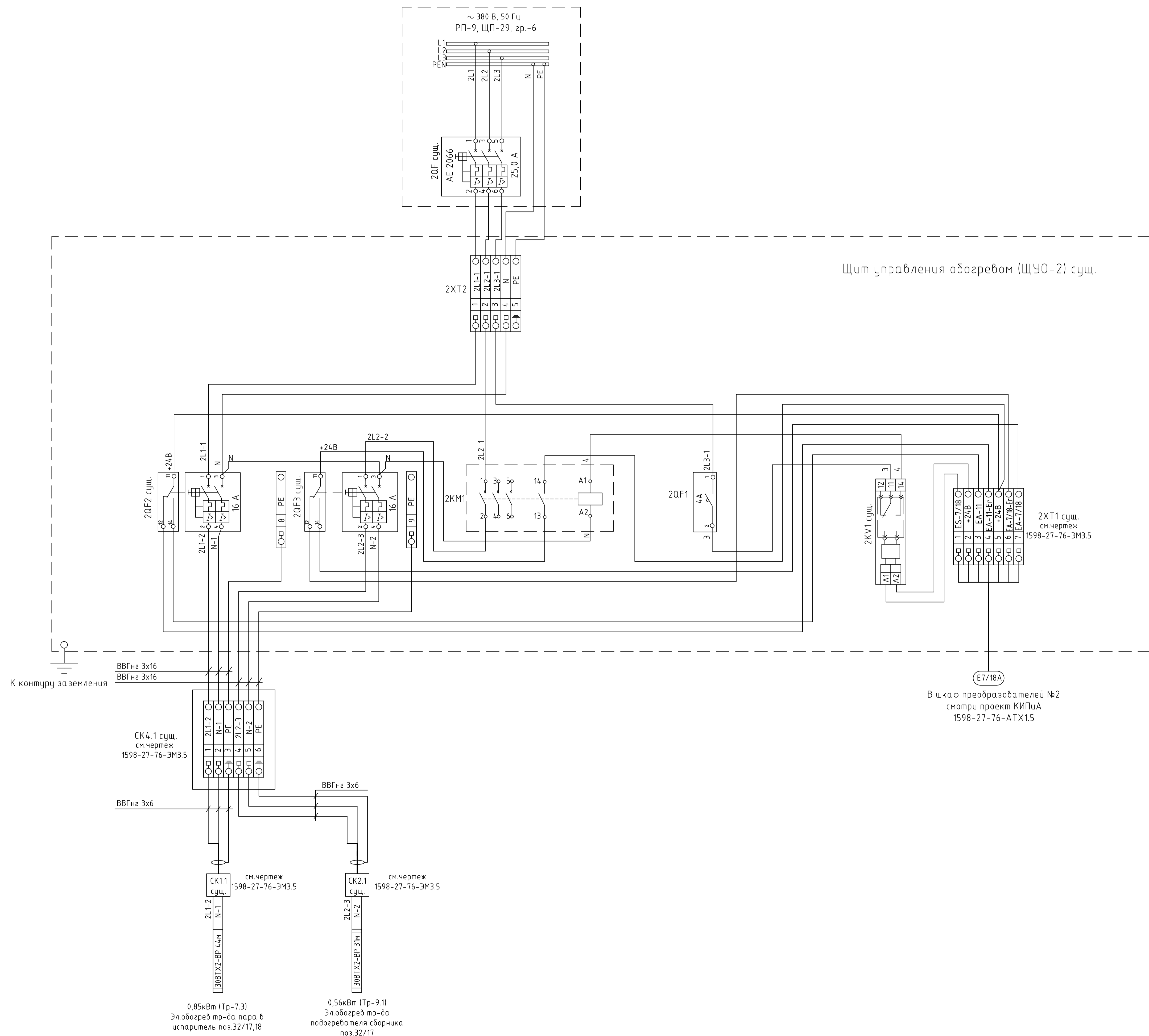
Схема подключений и соединений управления обогревом (ЩУО-2)
