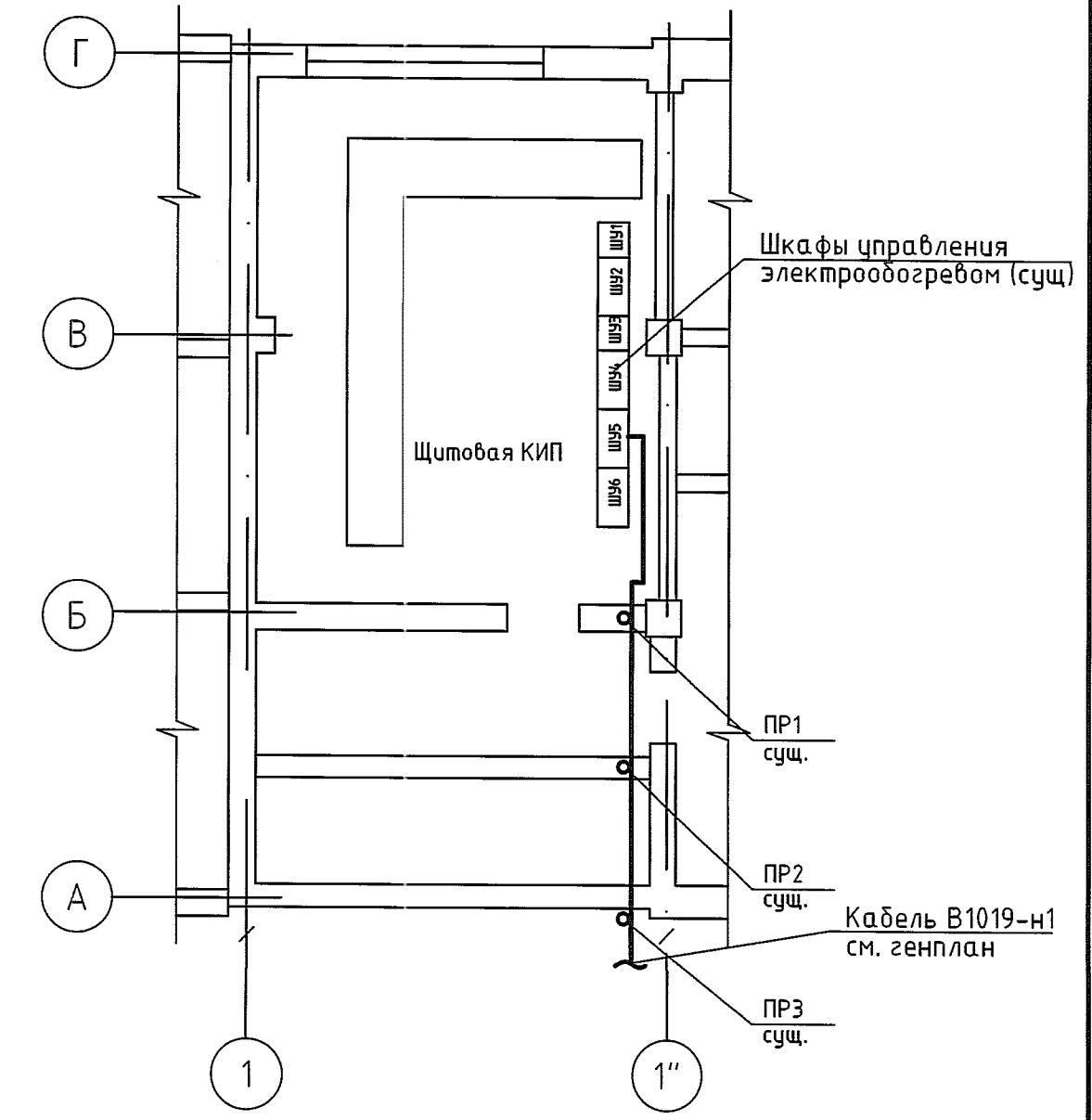
План к. 165 на отм. 0,000 (1:100)
