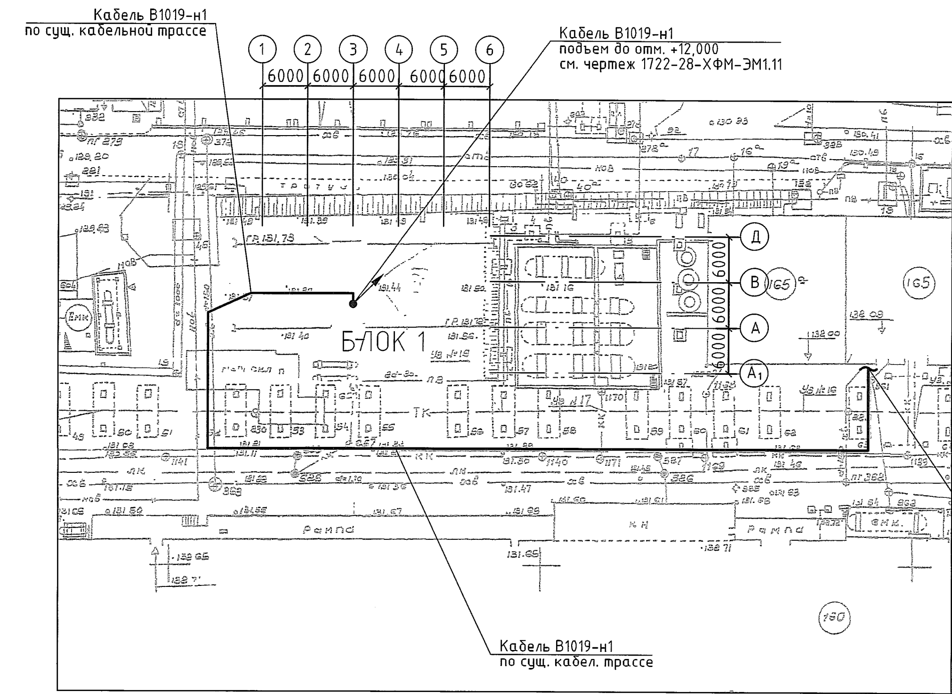
План трассы трубопроводов. Генплан. (1:500)
