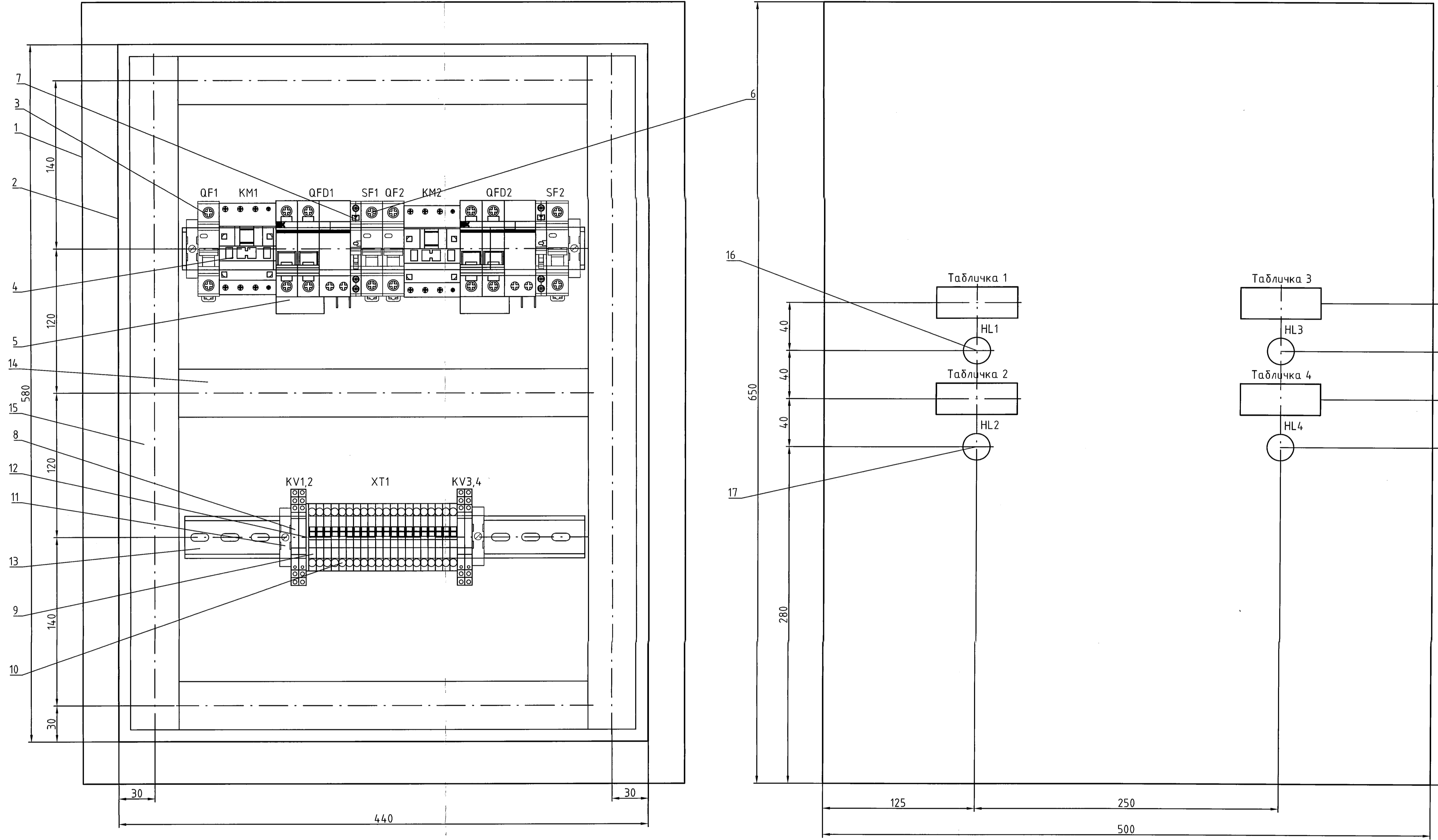
Шкаф управления электрообогревом (поз.ШУЭО) (1:2)
