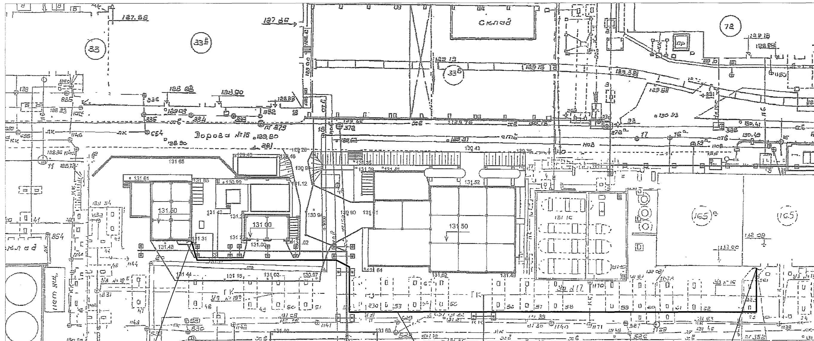
План трассы трубопроводов. Генплан. (1:500)
