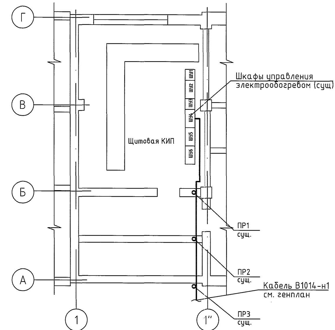
План к. 165 на отм. 0,000 (1:100)
